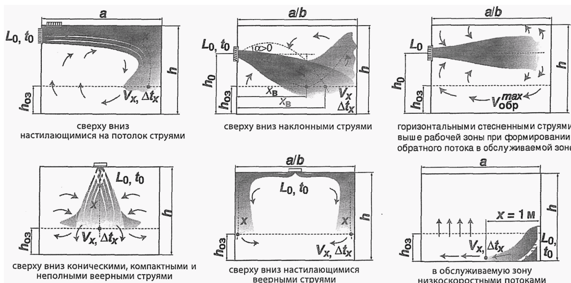
Рисунок Л.1 - Основные схемы подачи приточного воздуха
